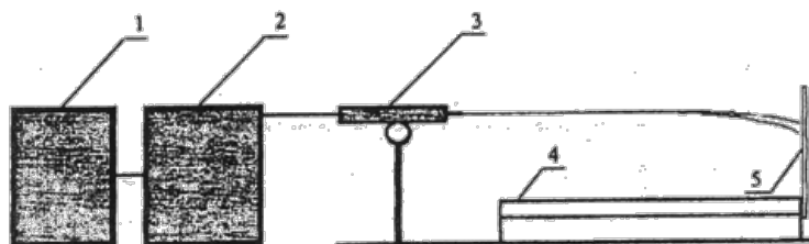
Рисунок 4. Схема установки для определения времени тушения горячей жидкости при подаче пены низкой кратности в борт противня:
