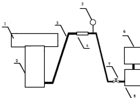
Рисунок 7. Схема установки для определения времени тушения горячей жидкости при подаче пены низкой кратности под слой нефтепродукта:
