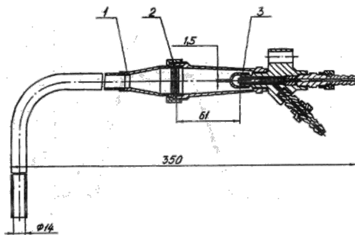
Рисунок 6. Генератор пены средней кратности по п.5.4 ГОСТ Р 50588:
