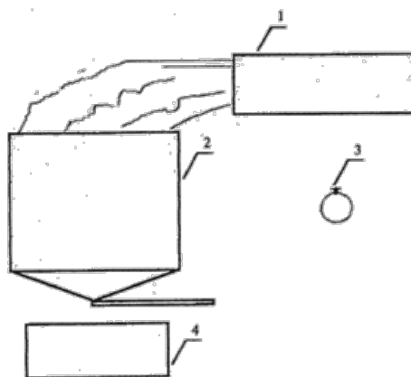
Рисунок 3. Схема установки для определения кратности и устойчивости пены высокой кратности:
