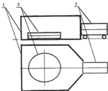
Рисунок 5. Схема установки для определения времени тушения горячей жидкости пеной высокой кратности:
