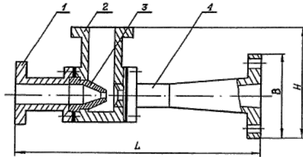
Рис. 1. Дозатор:
