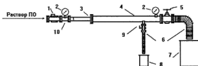
Рис. 1. Схема установки для испытания высоконапорных генераторов:
