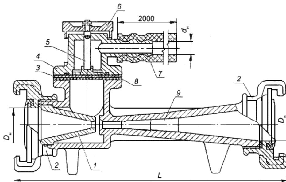
Рисунок А1 - Пеносмеситель ПС
